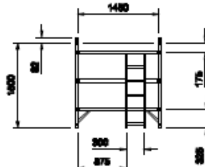
1.5m 3-Rung
