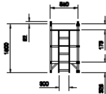
1.5m 3-Rung
